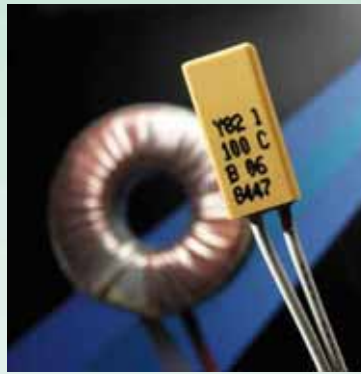
Tipo Y limitador Tª y corriente con R serie 0.12Alcc10.2A, VDE/UL Salida cable, c.i. y a medida.
