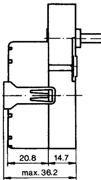
Motor mounting UDS 1..M
