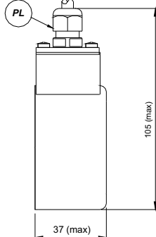
Pressacavo plastico elettroniche S/OC/P/OP/PP/PP2
