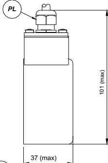
Pressacavo metallico per elettroniche LD / LD2
