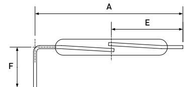
c) cut & bent
