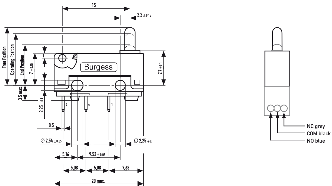
Dimensions
