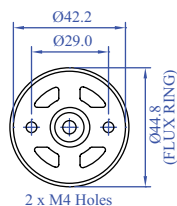
2 x M4 Holes
